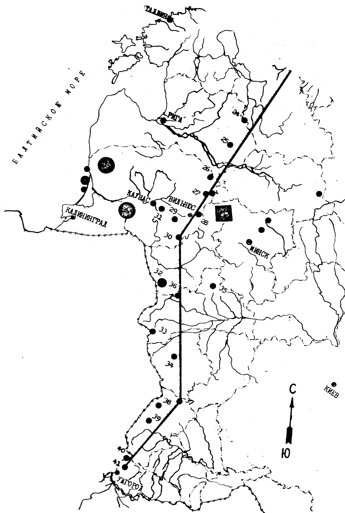
Рис. 6. Дендрохронологический профиль Мурманск-Карпаты (полная часть).
