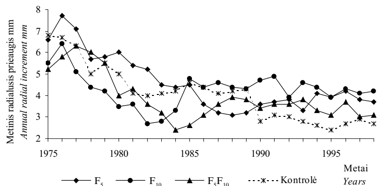
4 pav. Netradicinių mineralinių trąšų poveikis pušų radialiajam prieaugiui: F_5 – fosfogipsas 5 t/ha; F_{10} – fosfogipsas 10 t/ha; F_5P_{100} – fosfogipso 5 t/ha mišinys su superfosfatu 100 kg/ha fosforo veikliosios medžiagos; patręšta 1990 metais
