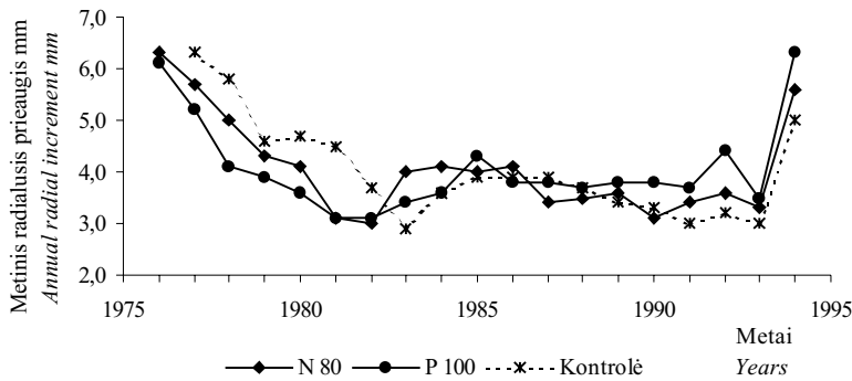
3 pav. Azoto ( N_{80} – karbamidas, 80 kg/ha azoto veikliosios medžiagos) ir fosforo ( P_{100} – superfosfatas, 100 kg/ha fosforo veikliosios medžiagos) trąšų poveikis pušų metiniam radialiajam prieaugiui; patręšta 1990 metais Fig. 3. Impact of nitrogen ( N_{80} – carbamide, 80 kg/ha of nitrogen active substance) and phosphorus ( P_{100} – superphosphate, 100 kg/ha phosphorus active substance) fertilizers on pine radial increment; fertilization year 1990
