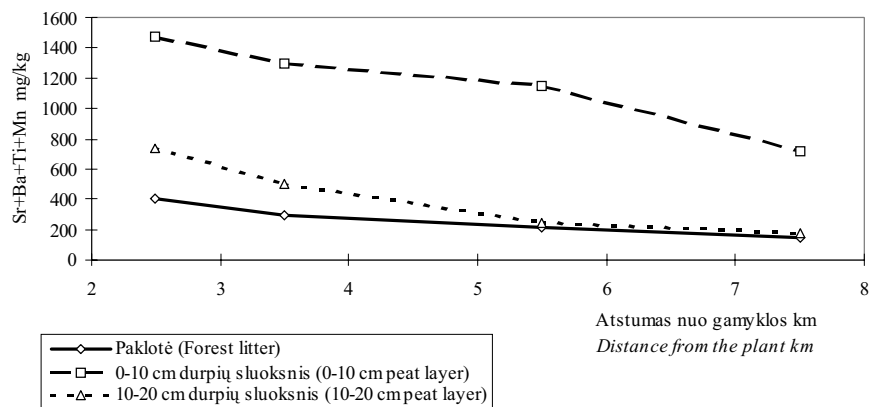
1 pav. „Akmenės cemento“ gamyklos emisijų poveikis stroncio, bario, titano ir mangano kiekių sumai durpiniame dirvožemyje
