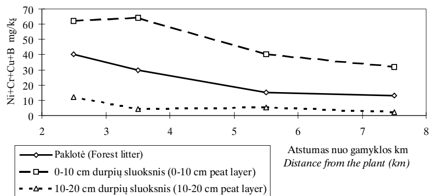
2 pav. „Akmenės cemento“ gamyklos emisijų poveikis nikelio, chromo, vario ir boro kiekių sumai durpiniame dirvožemyje
